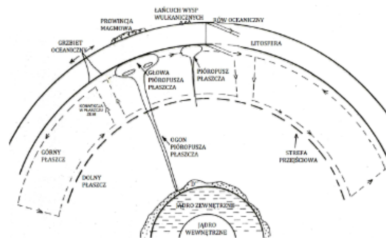
Ryc. 1. Schemat powstawania i przemieszczania strumienia płaszcza (opracowano na podstawie Raval i Veeraswamy, 2003)
